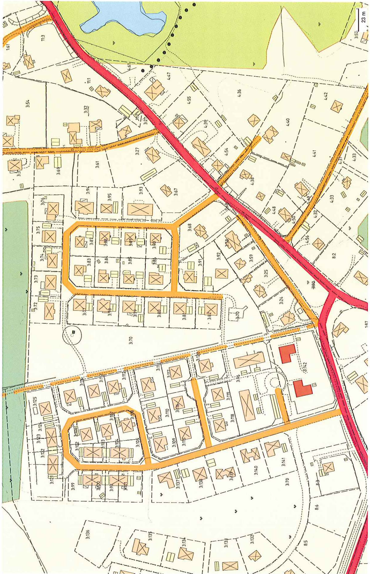
Autoka-Vy 3.0
